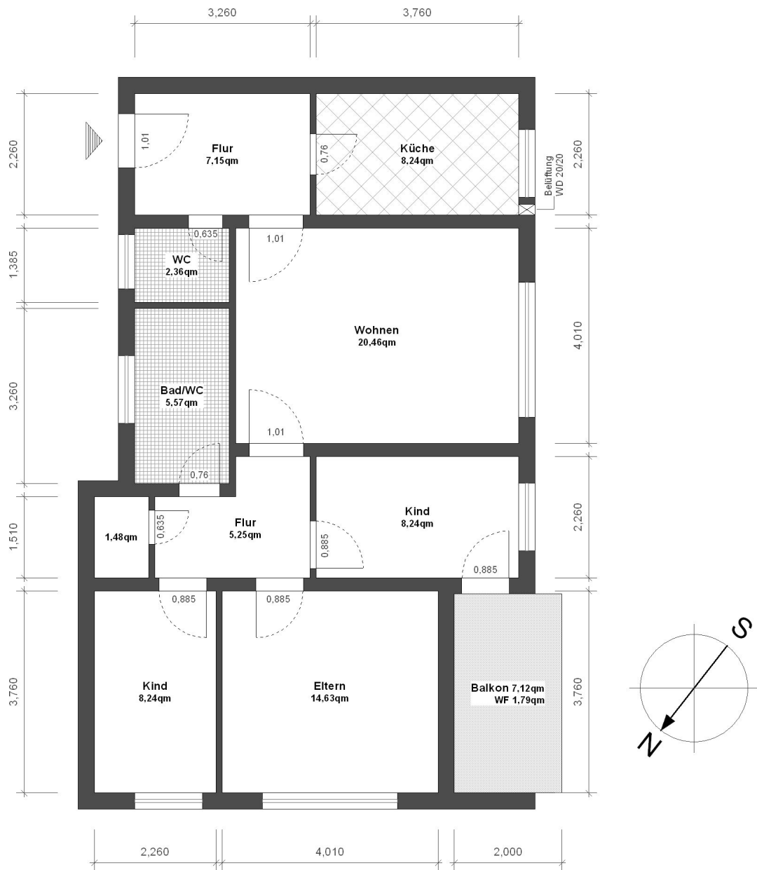
Wohnungstyp D - 84qm
